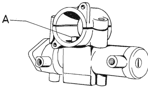
Abb. 36 Lenkradschloß, 120 A = Sperrzapfen
