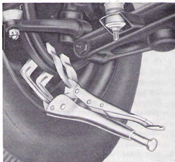
Abb. 7 Blockierung der Bremstrommel
