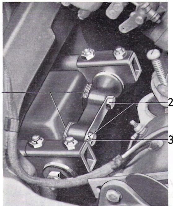
Abb. 8 Einstellvorrichtung für Sturz und Nachlauf, Querlenkerachse – Vorderachsträger
