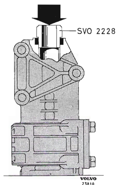
Abb. 51. Einbau der Lagerbuchse, Lenkrolle
