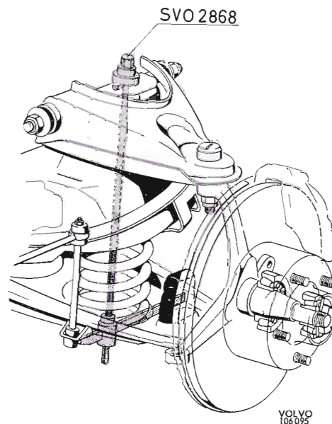
Abb. 16 Zusammenpressen der Feder
