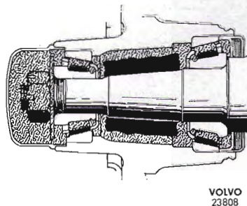
Abb. 23 Fett im Vorderradlager
