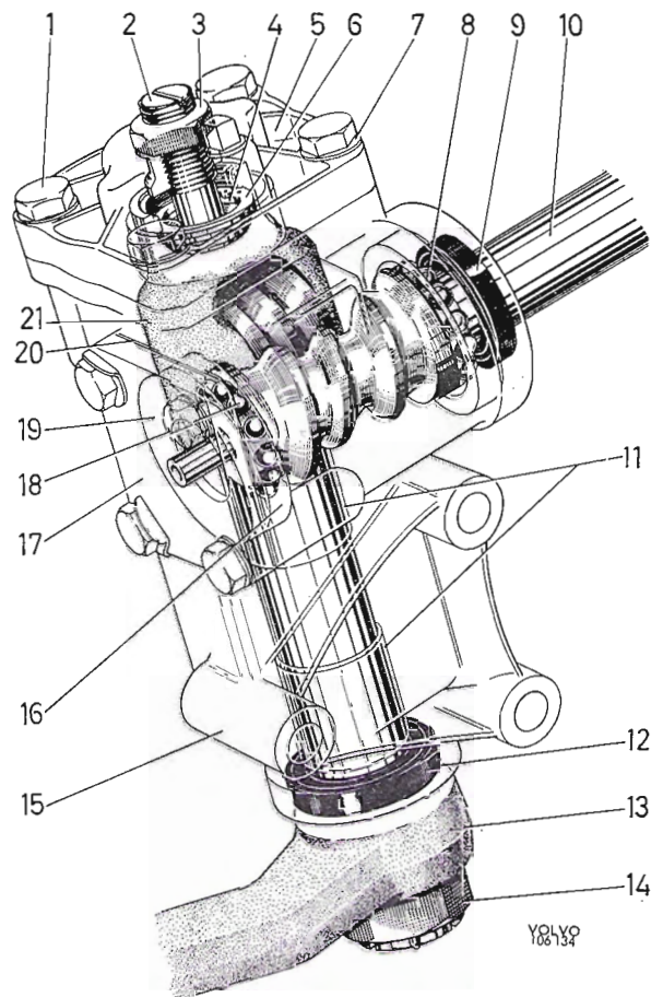
Abb. 37 Lenkgetriebe
