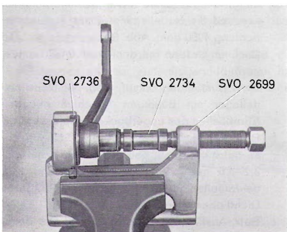
Abb. 65 Ausbau der Buchse im Umlenkhebel
