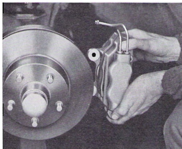
Abb. 19 Ausbau des Bremsattels, früh. Ausf.
