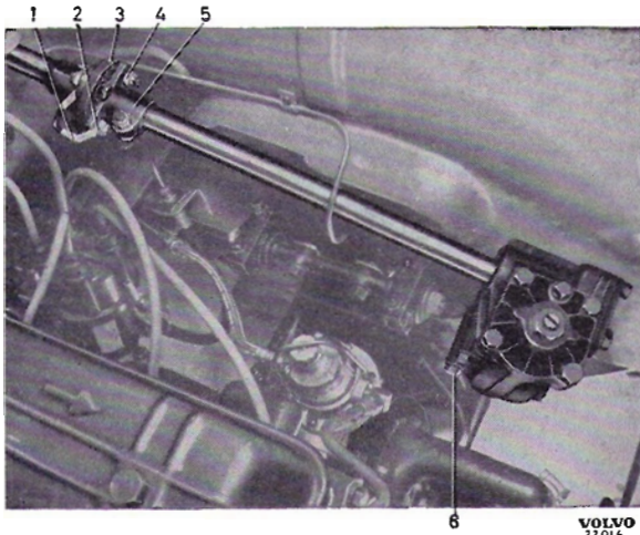
Abb. 46 Lenkgetriebe, 120 früh. Ausf.
