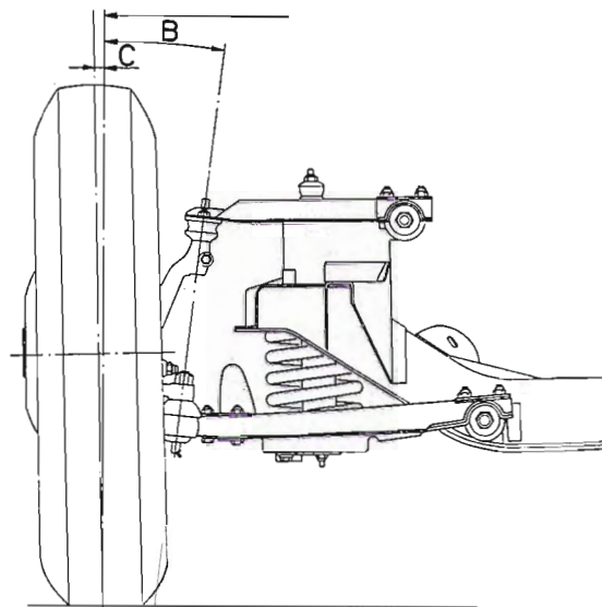
Abb. 5 Sturz und Spreizung
