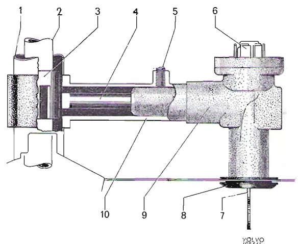
Abb. 45 Lenkradschloß, 1800
