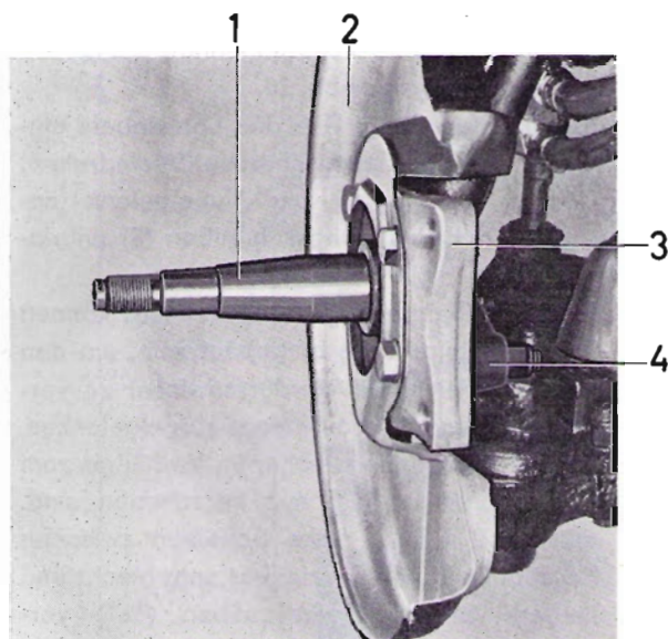
Abb. 24 Teile der Vorderachse und Radaufhängung
