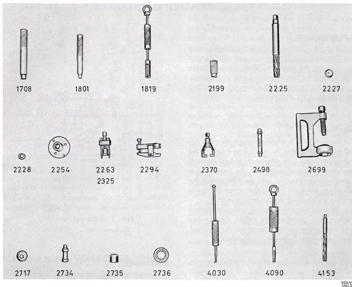
Abb. 3 Spezialwerkzeuge für Arbeiten an der Lenkvorrichtung
