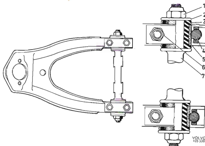
Abb. 14 Oberer Querlenker
