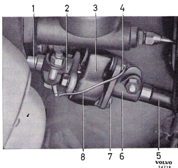
Abb. 58 Gummigelenkkupplung, 1800
