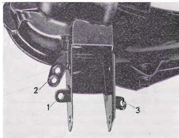
Abb. 17 Vorderachsträger
