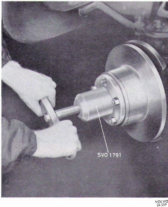
Abb. 21 Ausbau der Nabe
