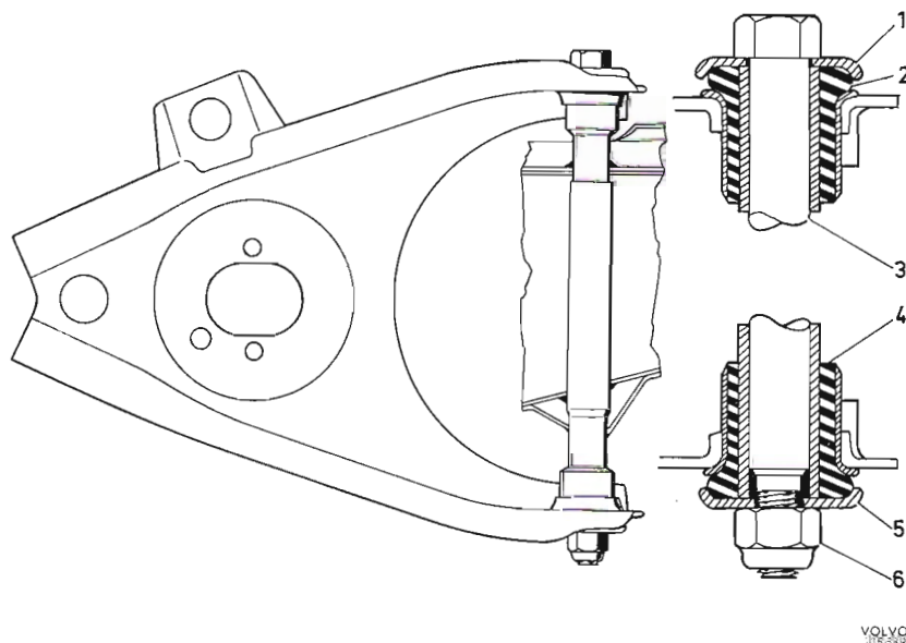
Abb. 15 Unterer Querlenker, spät. Ausf.
