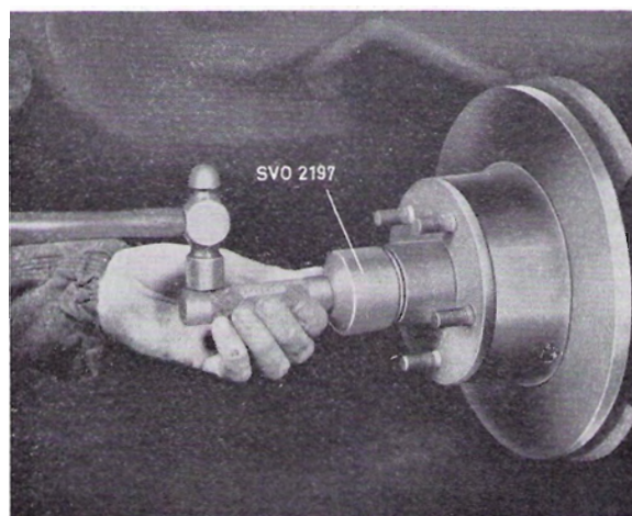
Abb. 20 Ausbau der Fettbüchse
