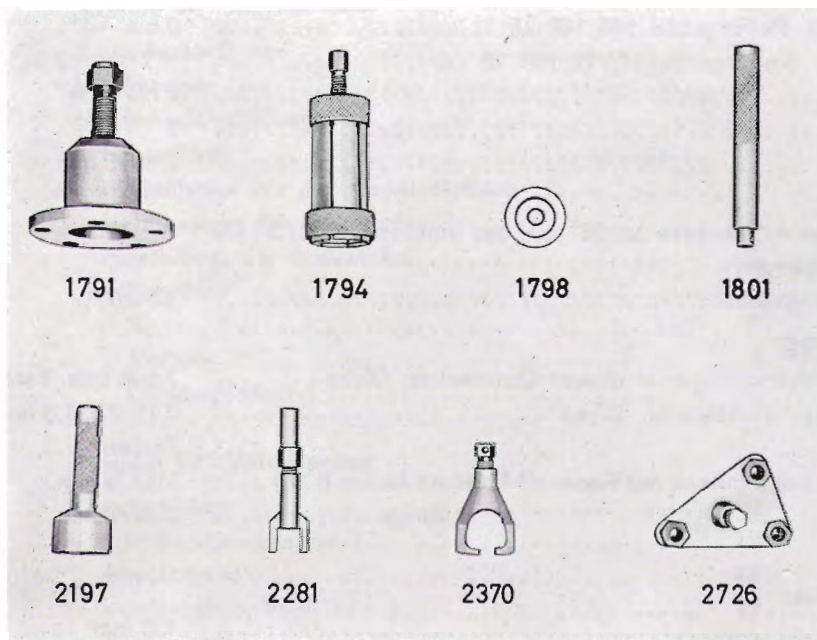
Abb. 1 Spezialwerkzeuge für Arbeiten an der Vorderachse
