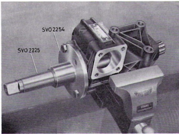
Abb. 52 Ausreiben der Lagerbuchsen, Lenkrolle
