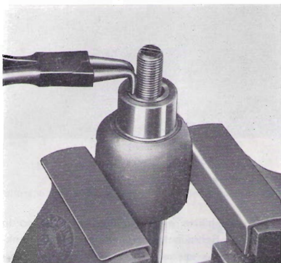
Abb. 49 Ausfedern der Innensicherung
