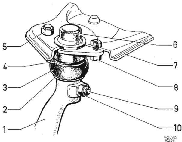
Abb. 26 Befestigung des oberen Kugelgelenkes
