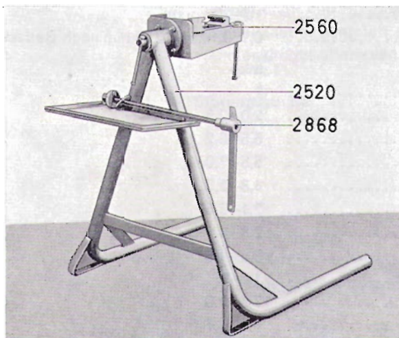
Abb. 2 Spezialwerkzeuge für Arbeiten an der ausgebauten Vorderachse
