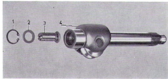
Abb. 54 Lenkrollenwelle
