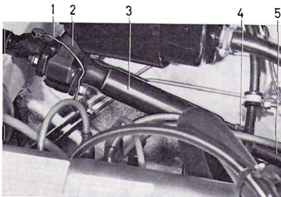
Abb. 47 Lenkungsteile, 1800 spät. Ausf.
