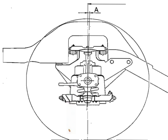
Abb. 4 Nachlauf
